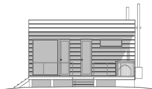
Julkisivu 1
